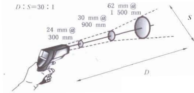
图 A.2 一种典型的测量距离与视场关系图 (D-S 图)
